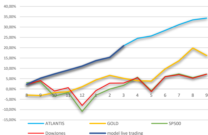
Benchmark table
